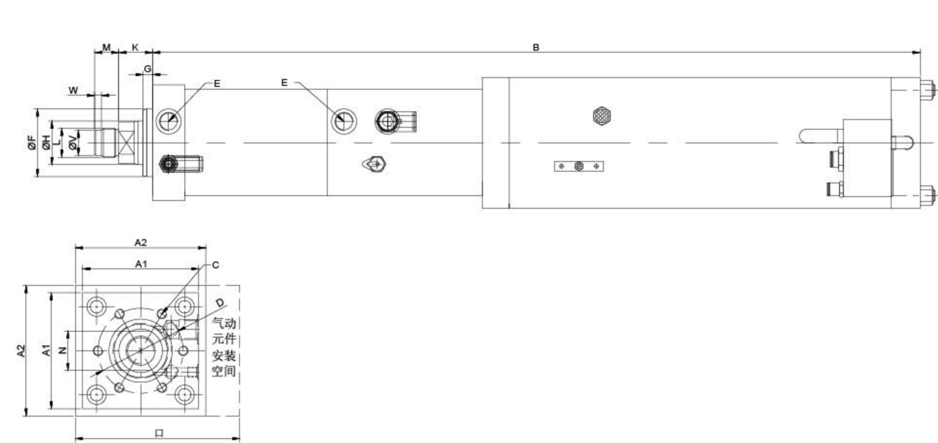
BS系列气液增力缸尺寸图
