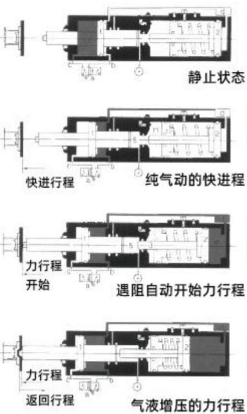
1 SIMITCH气液增压缸工作过程
