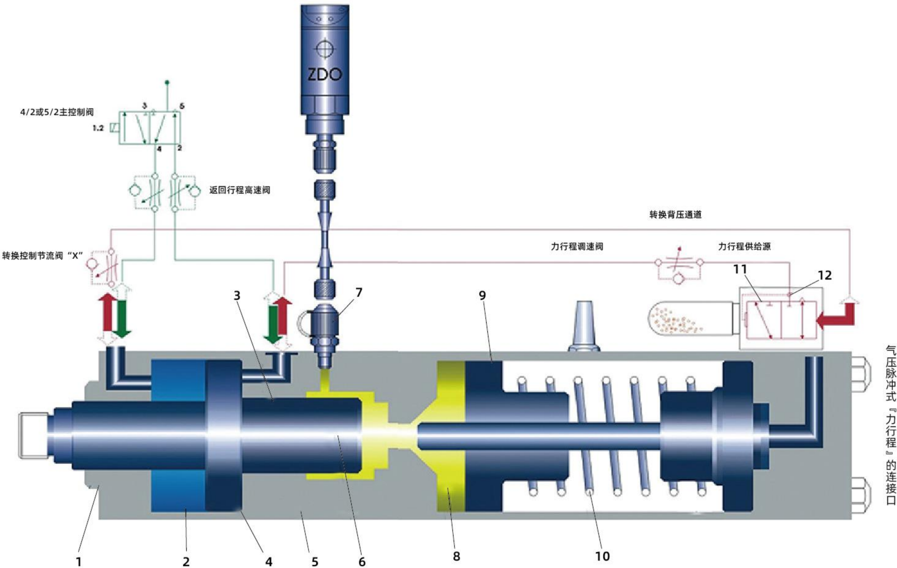
1 SIMITCH气液增压缸工作过程
